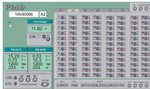
Panel virtual para control de un módulo de E/S de 6tl
