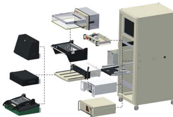
Módulos en rack 19" para integrar un sistema de test
