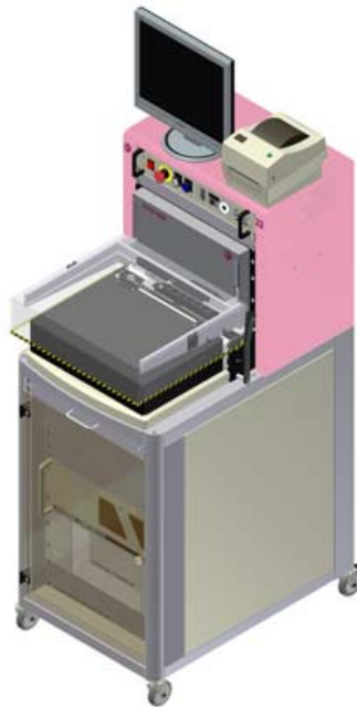
Plataforma de test 6tl-22, a partir de módulos controlados por CAN
